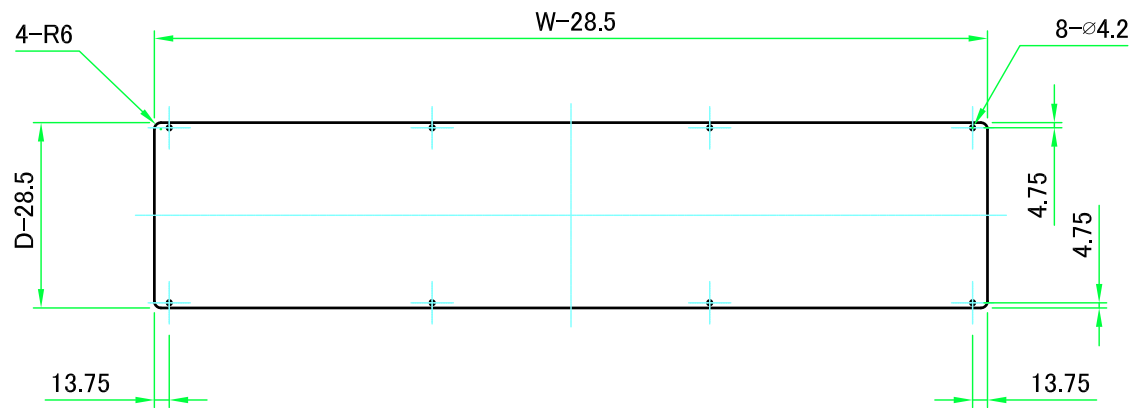
パネル裏面 / Panel Backside
